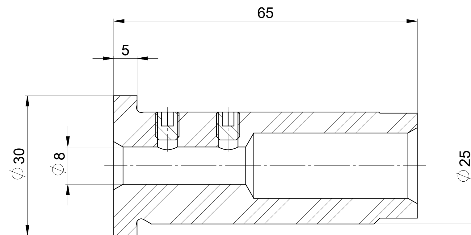
SEZIONE A-A
