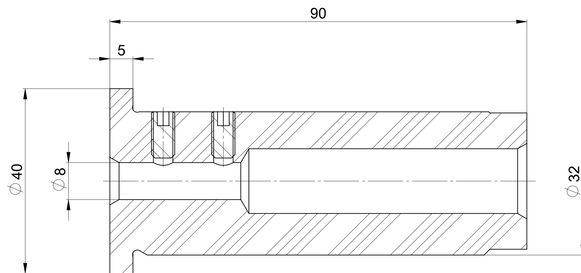
SEZIONE A-A
