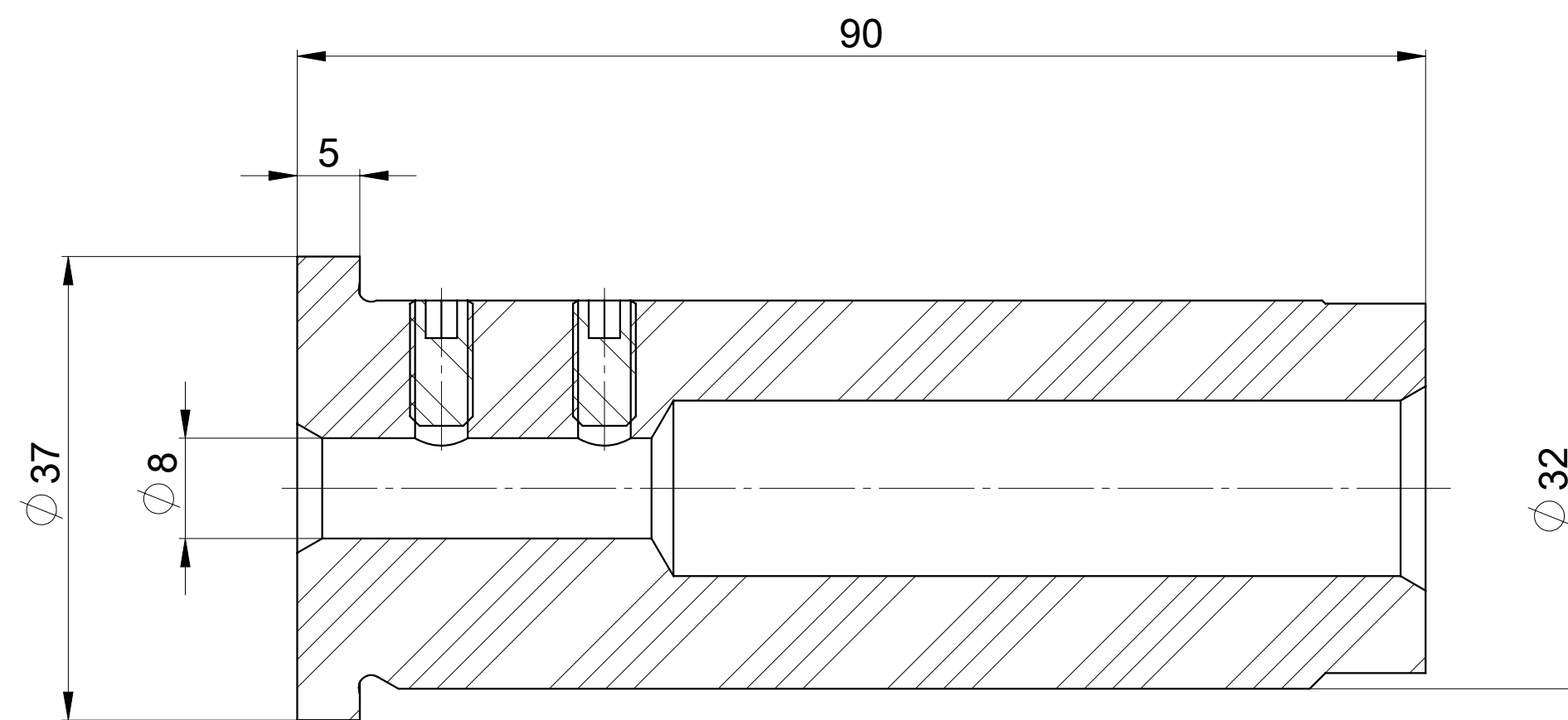
SEZIONE A-A
