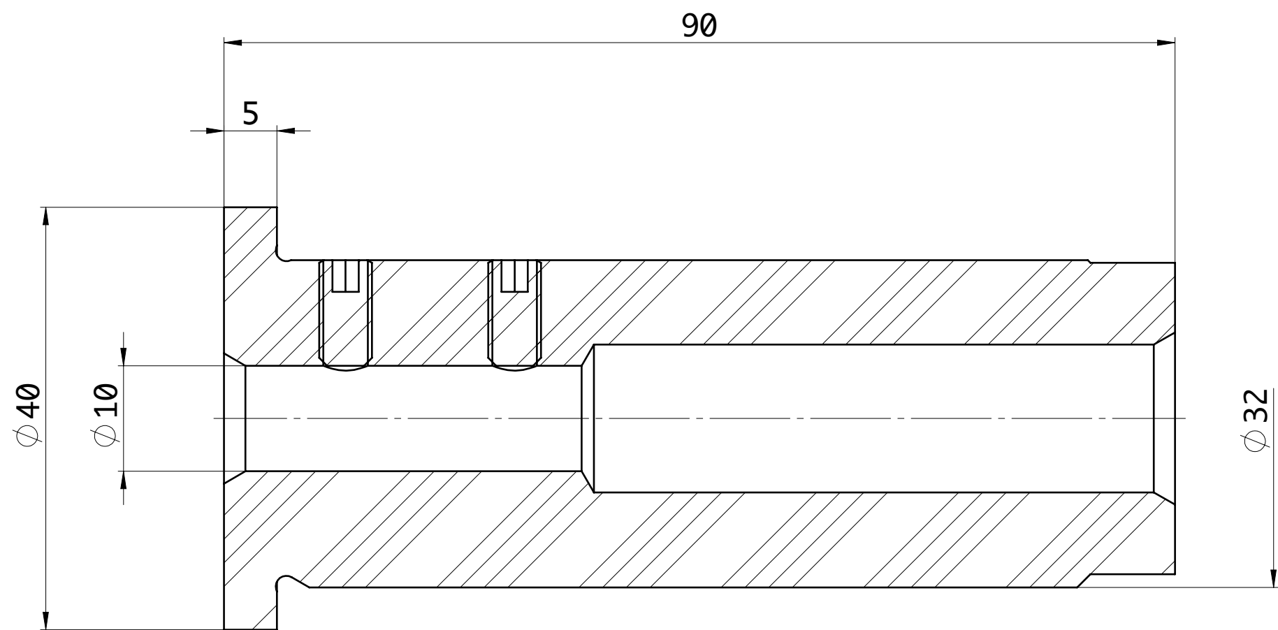
SEZIONE A-A
