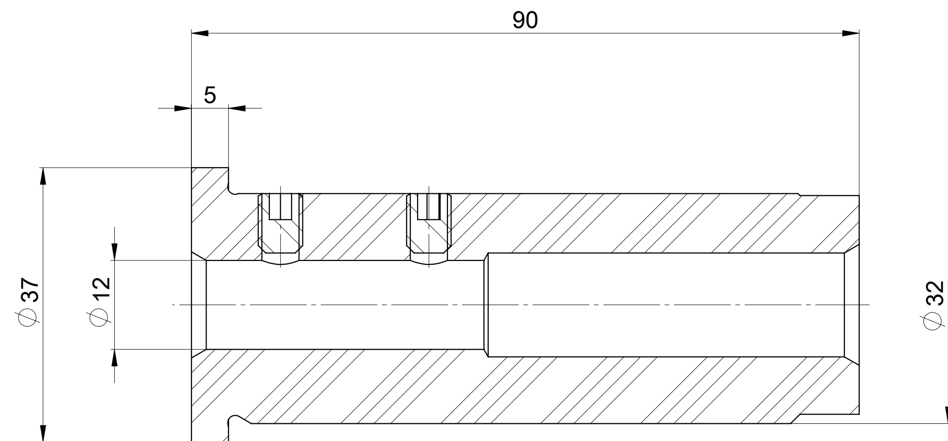
SEZIONE A-A
