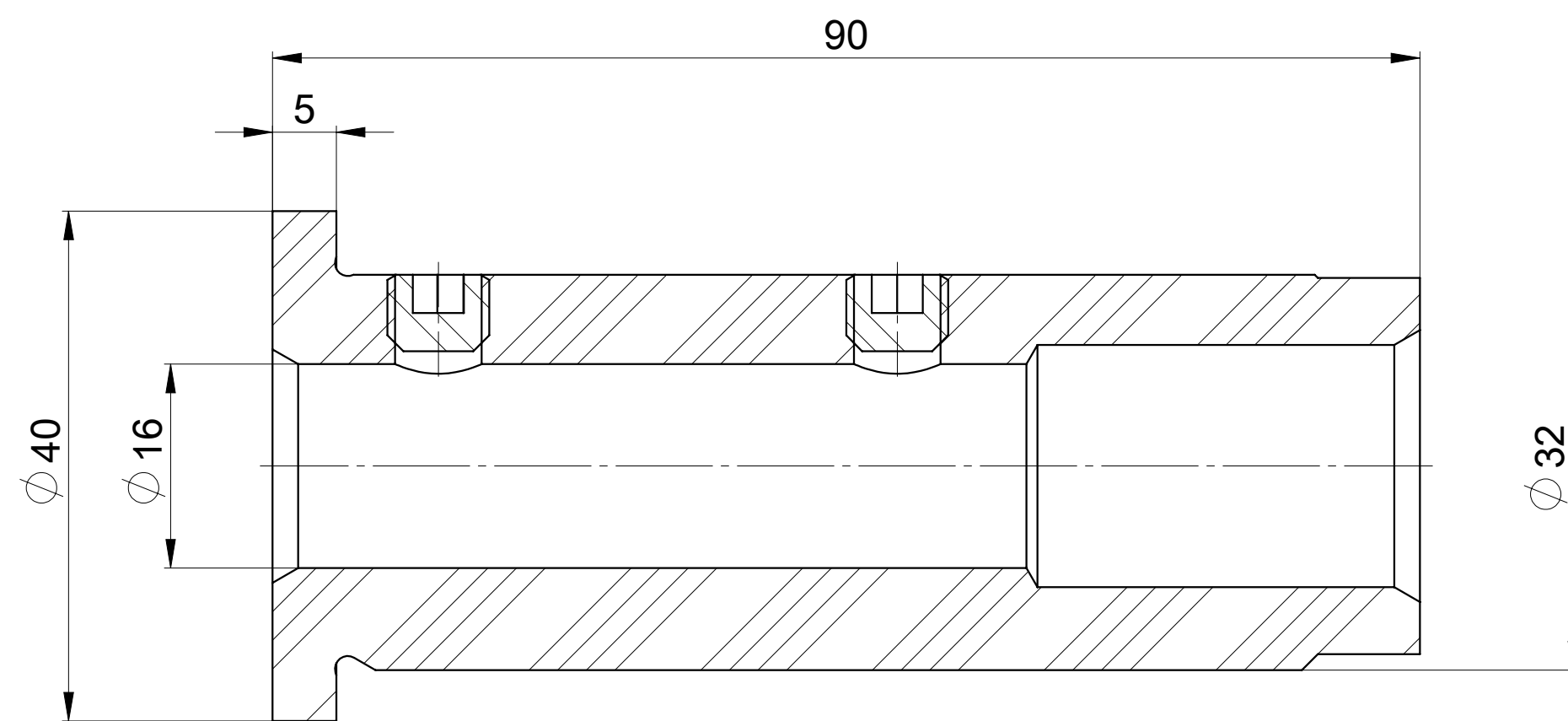
SEZIONE A-A
