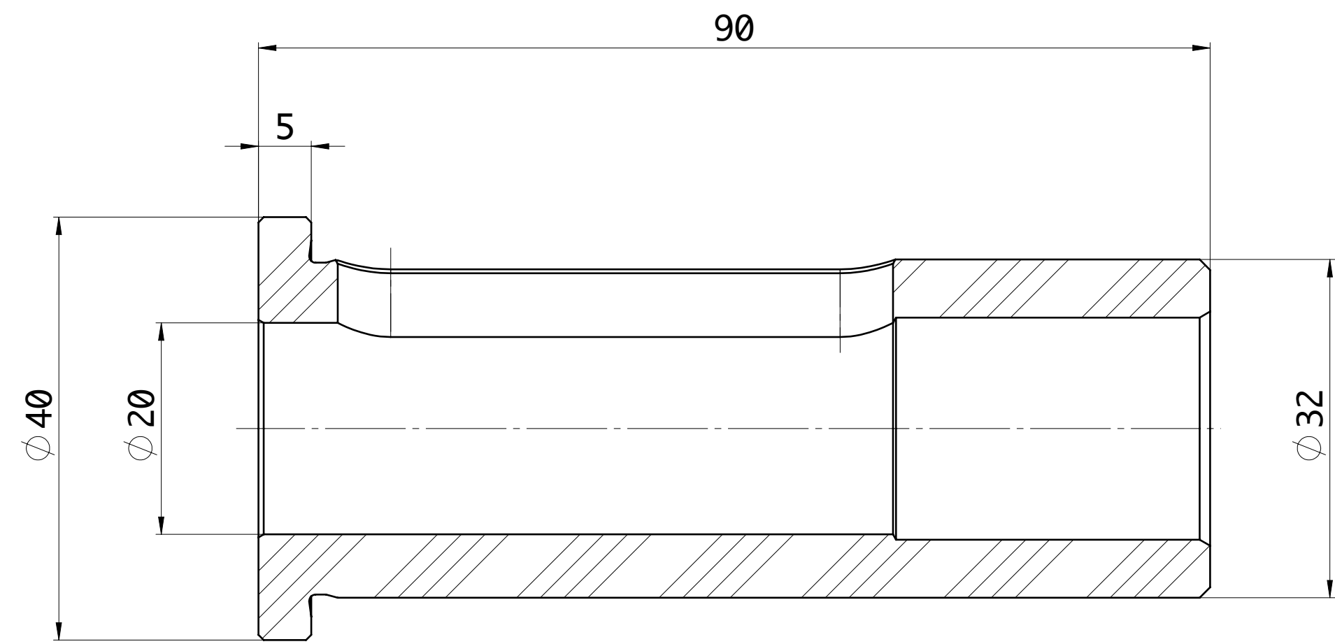
SEZIONE A-A
