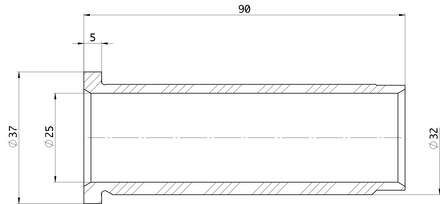
SEZIONE A-A
