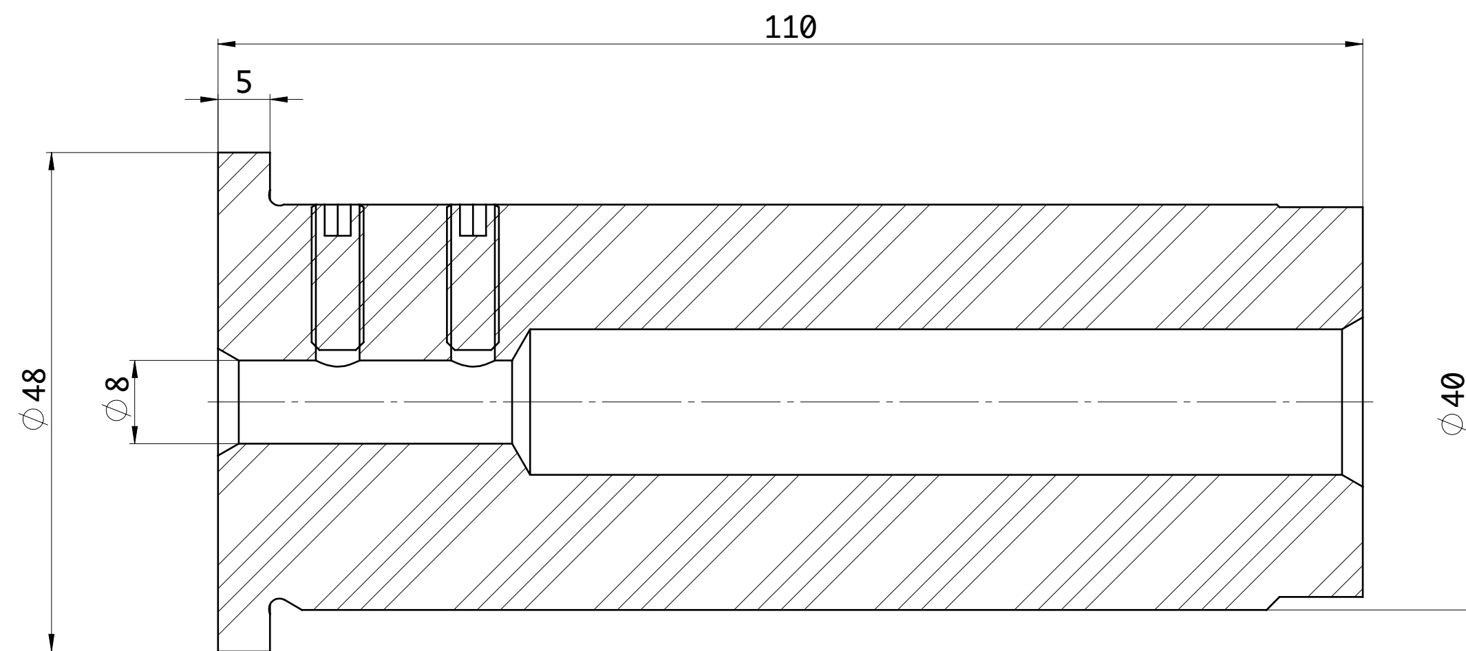
SEZIONE A-A
