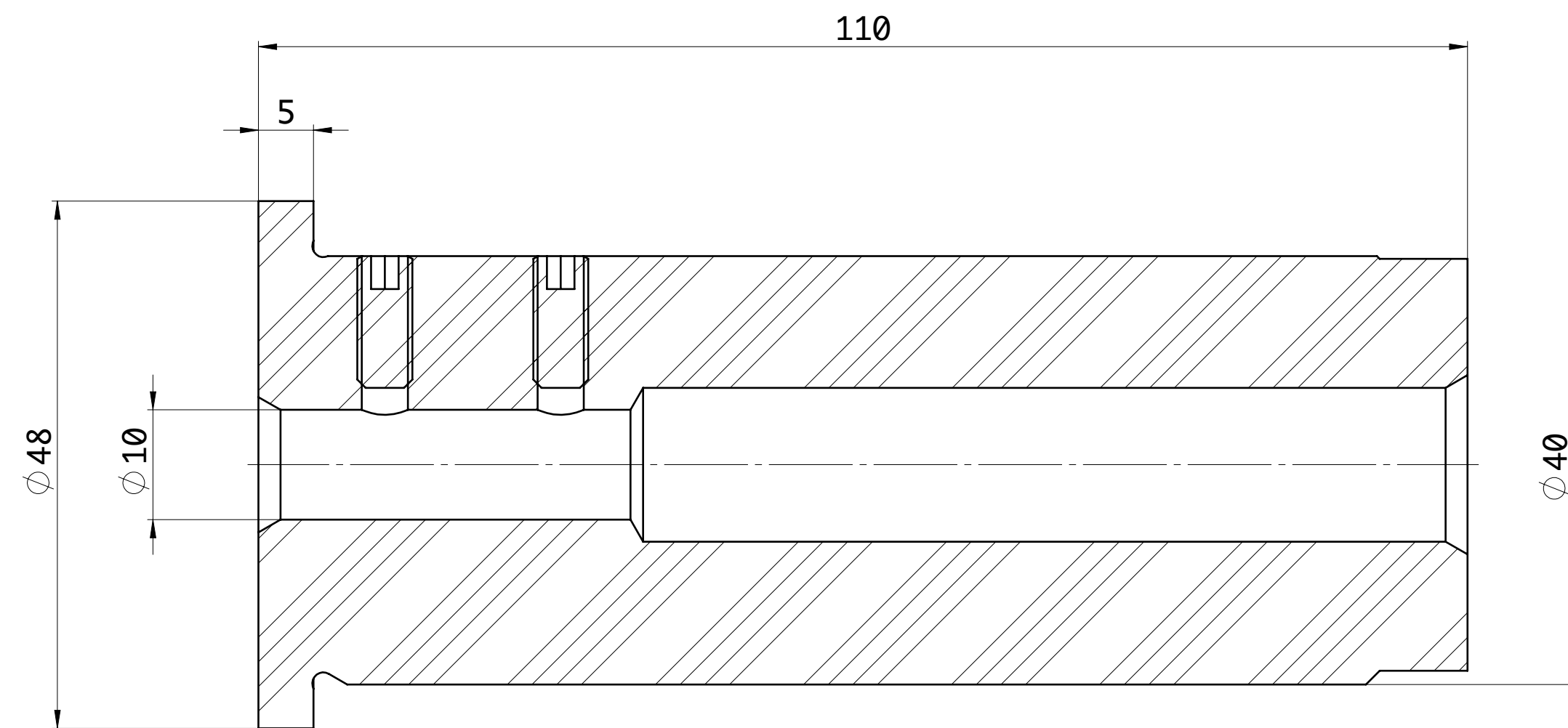
SEZIONE A-A
