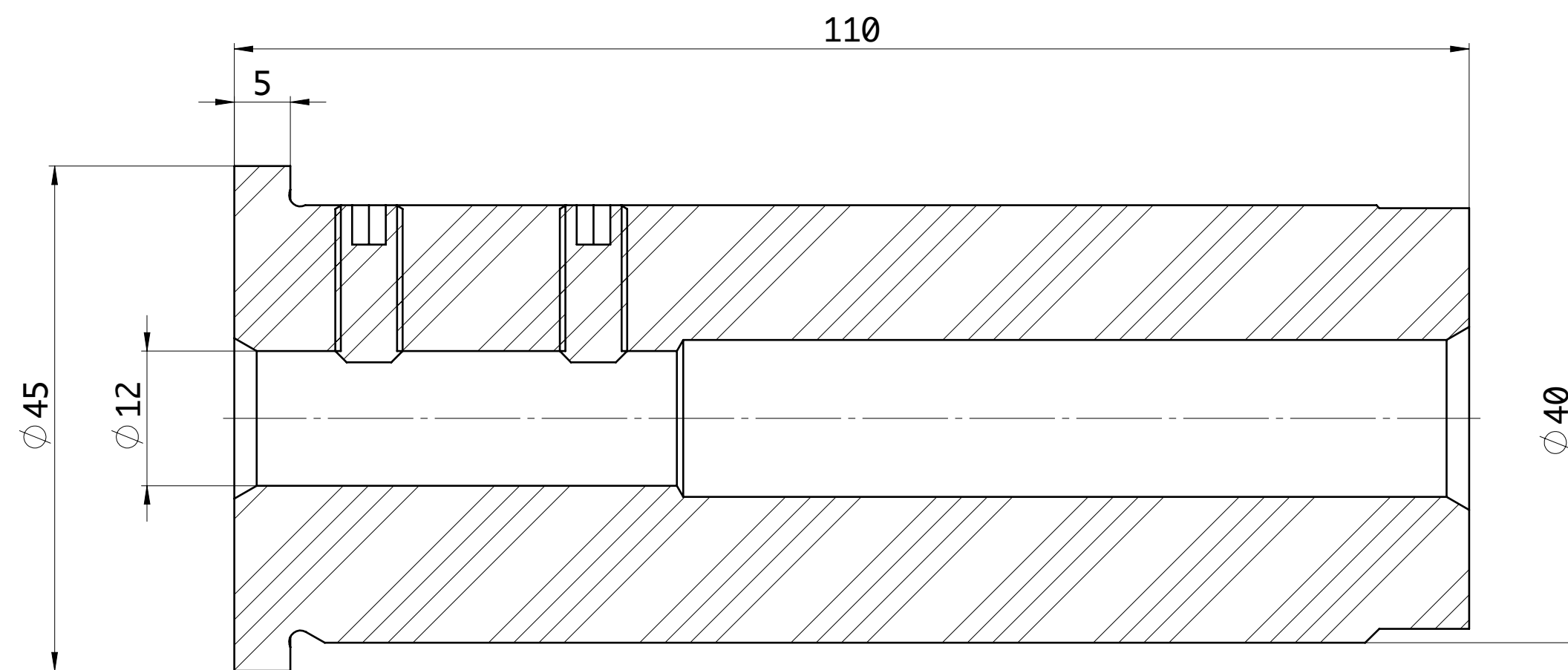
SEZIONE A-A
