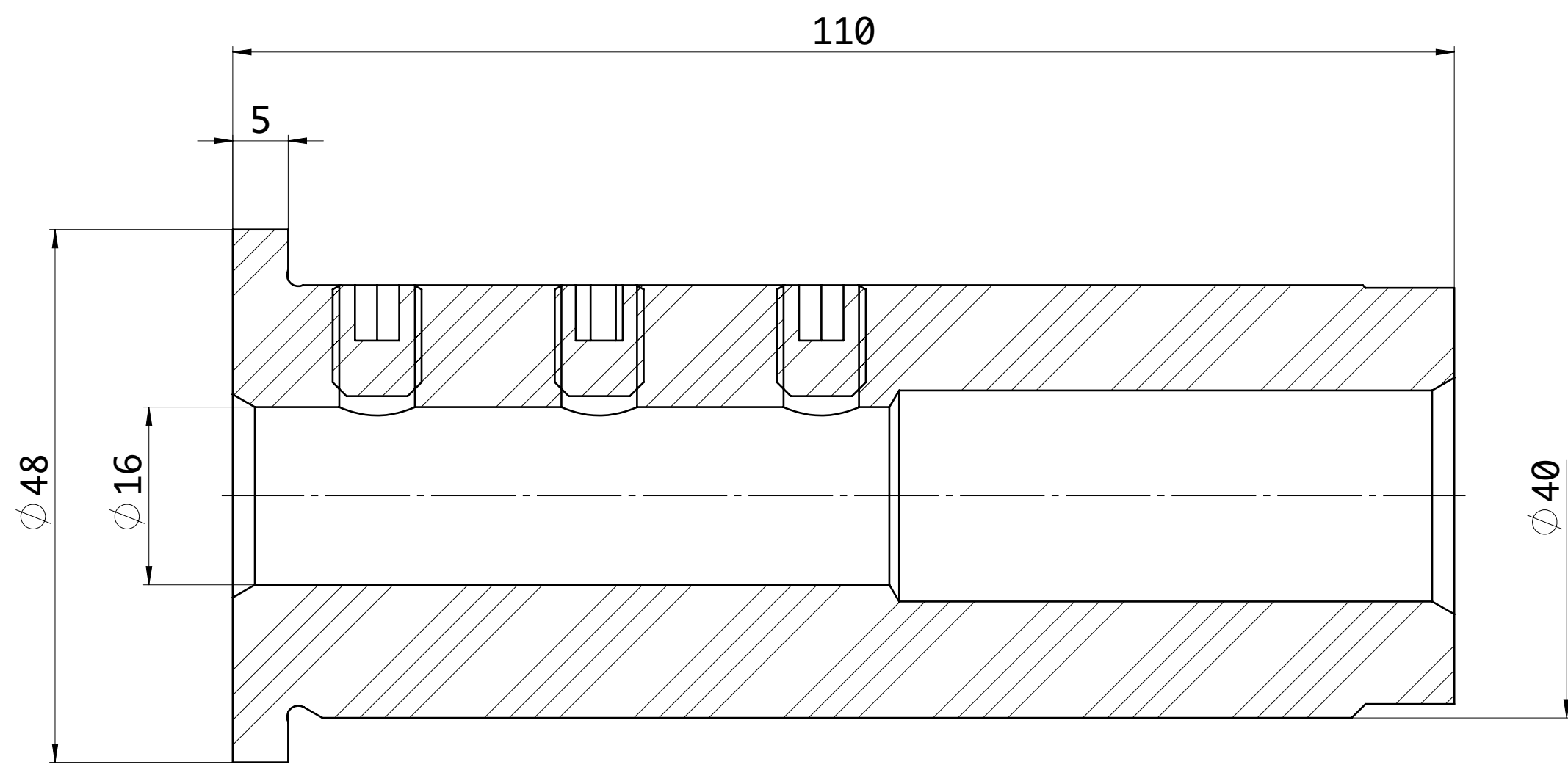
SEZIONE A-A
