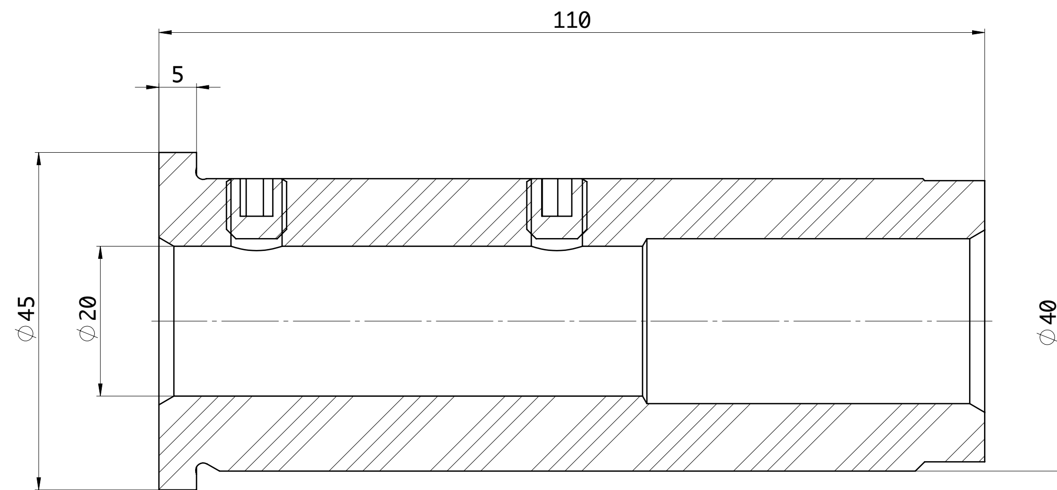
SEZIONE A-A
