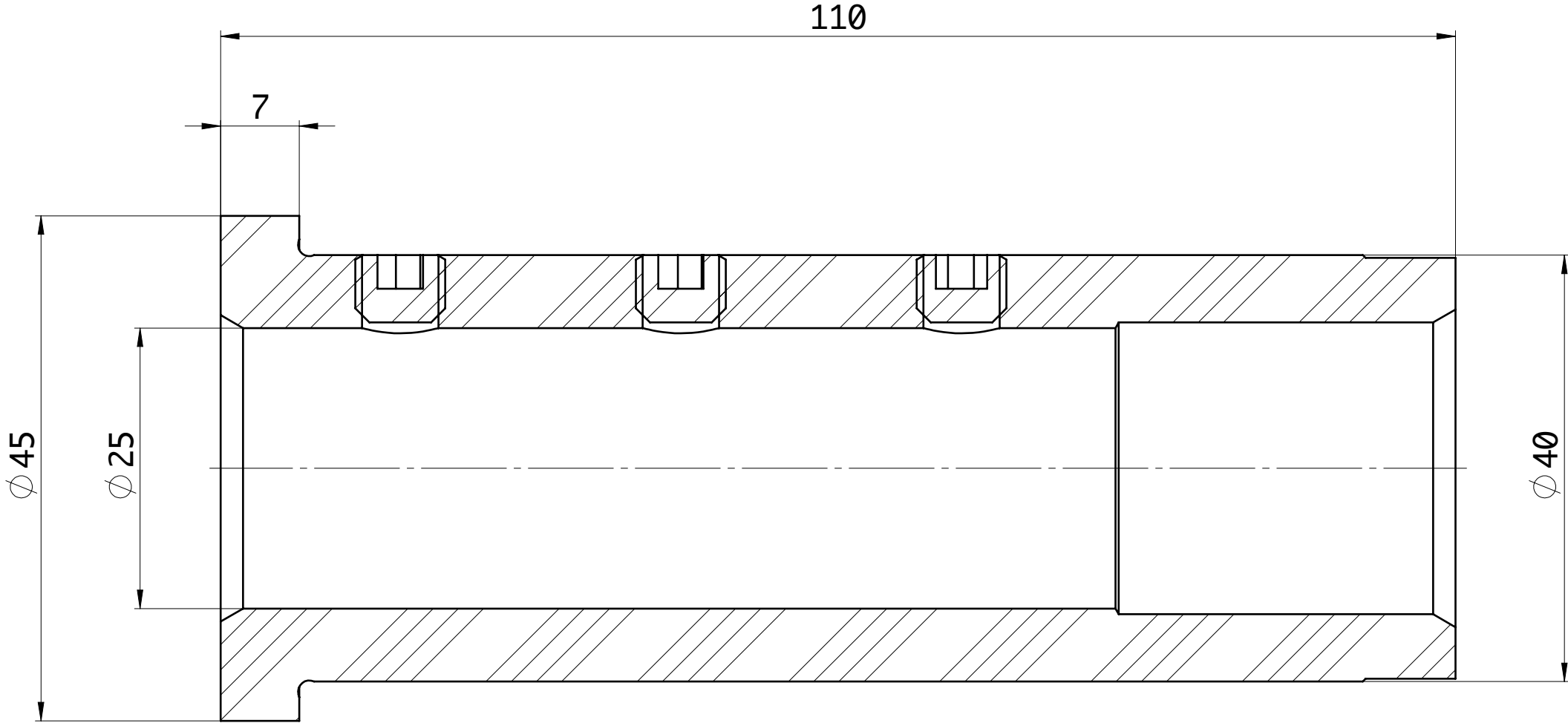
SEZIONE A-A
