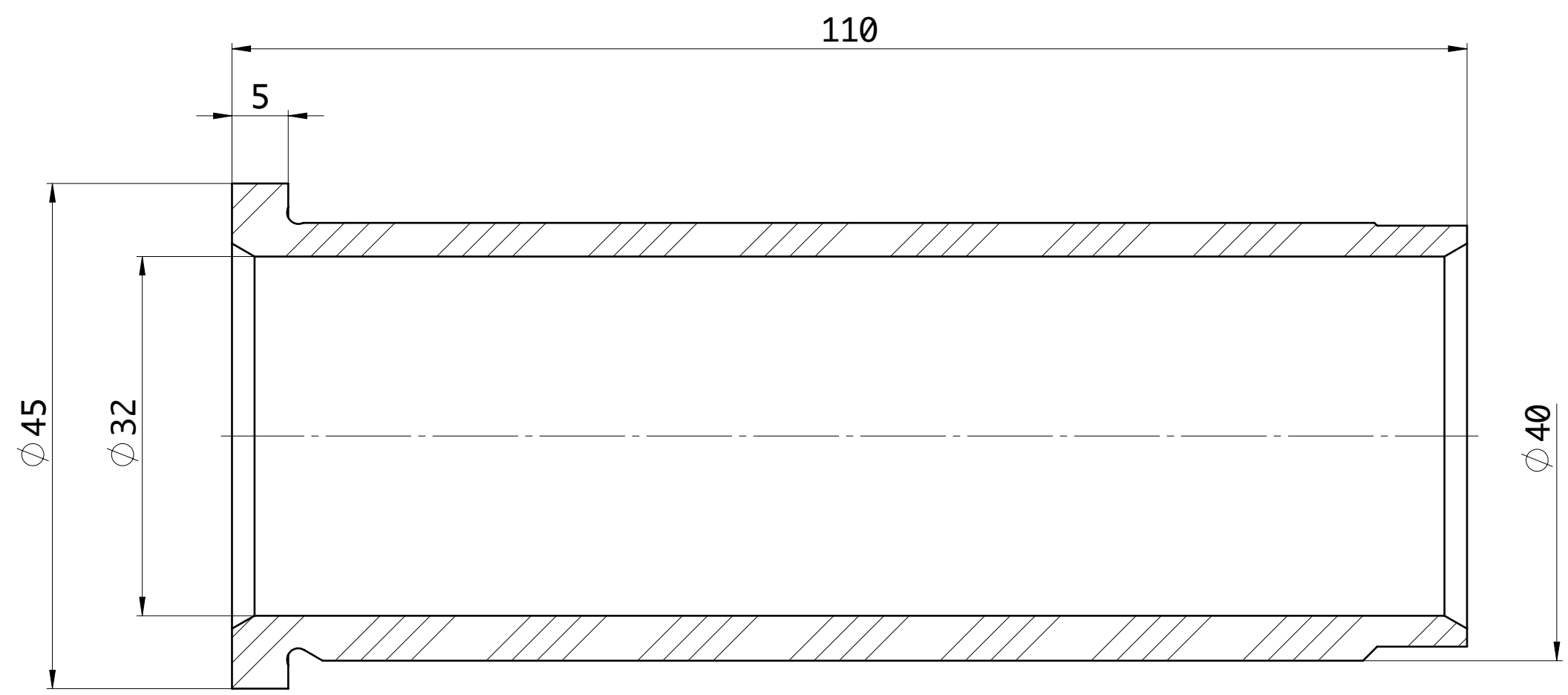
SEZIONE A-A
