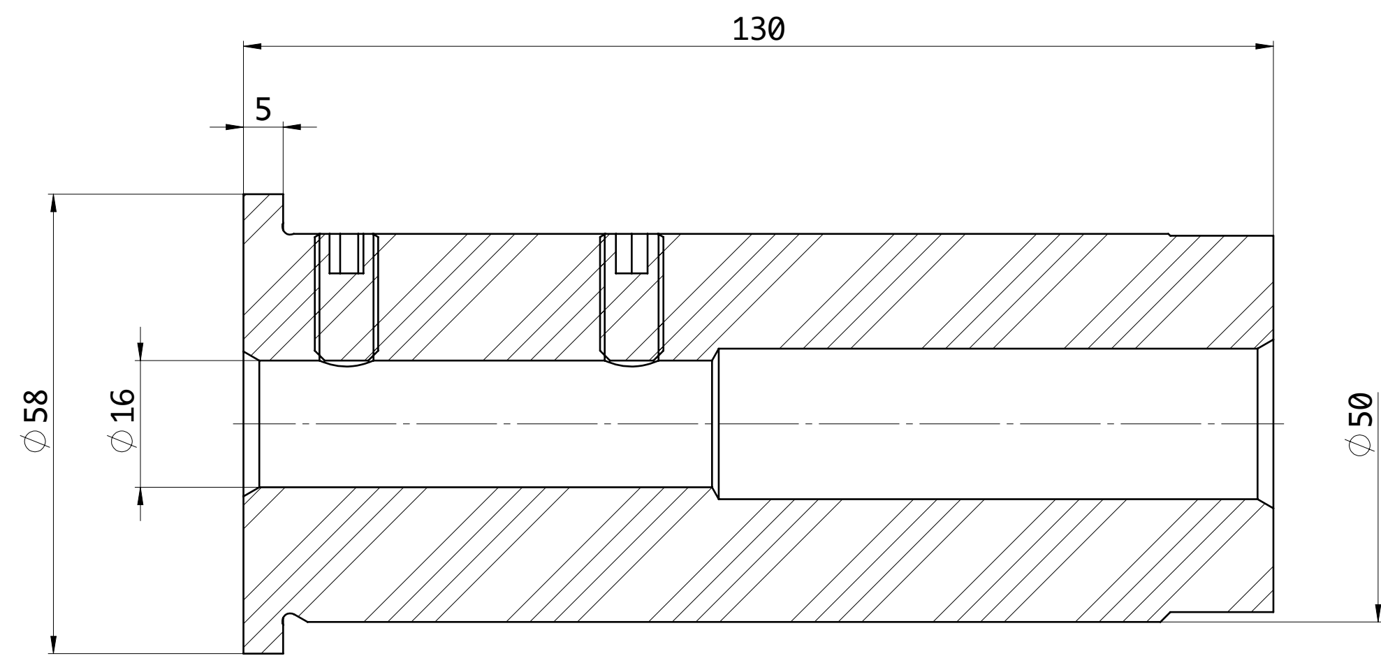
SEZIONE A-A
