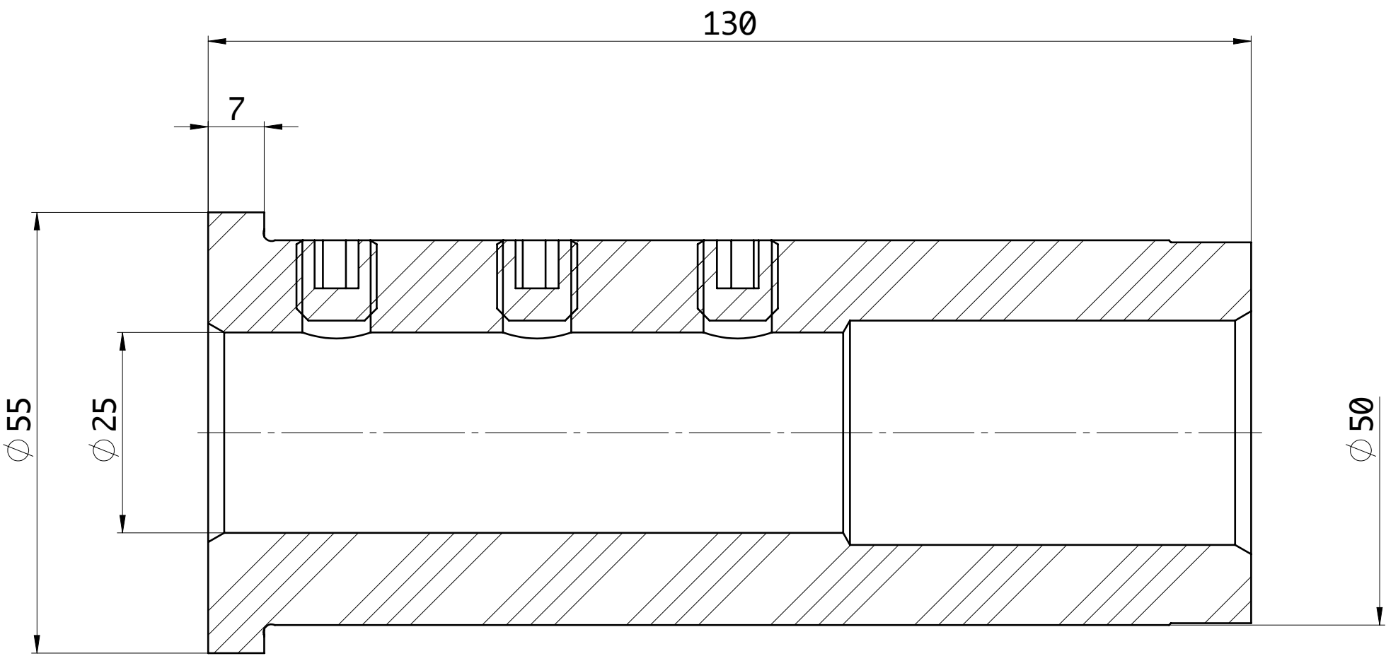
SEZIONE A-A
