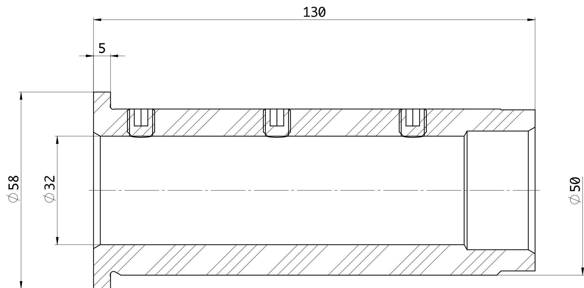
SEZIONE A-A
