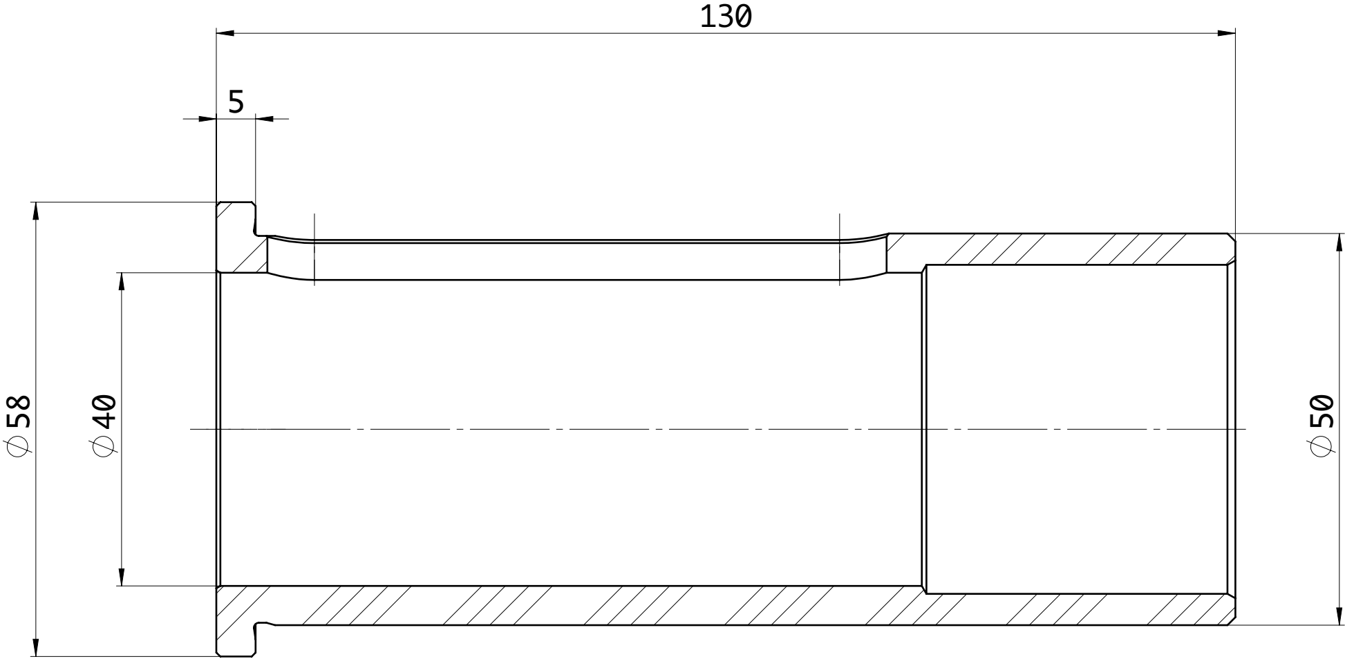
SEZIONE A-A
