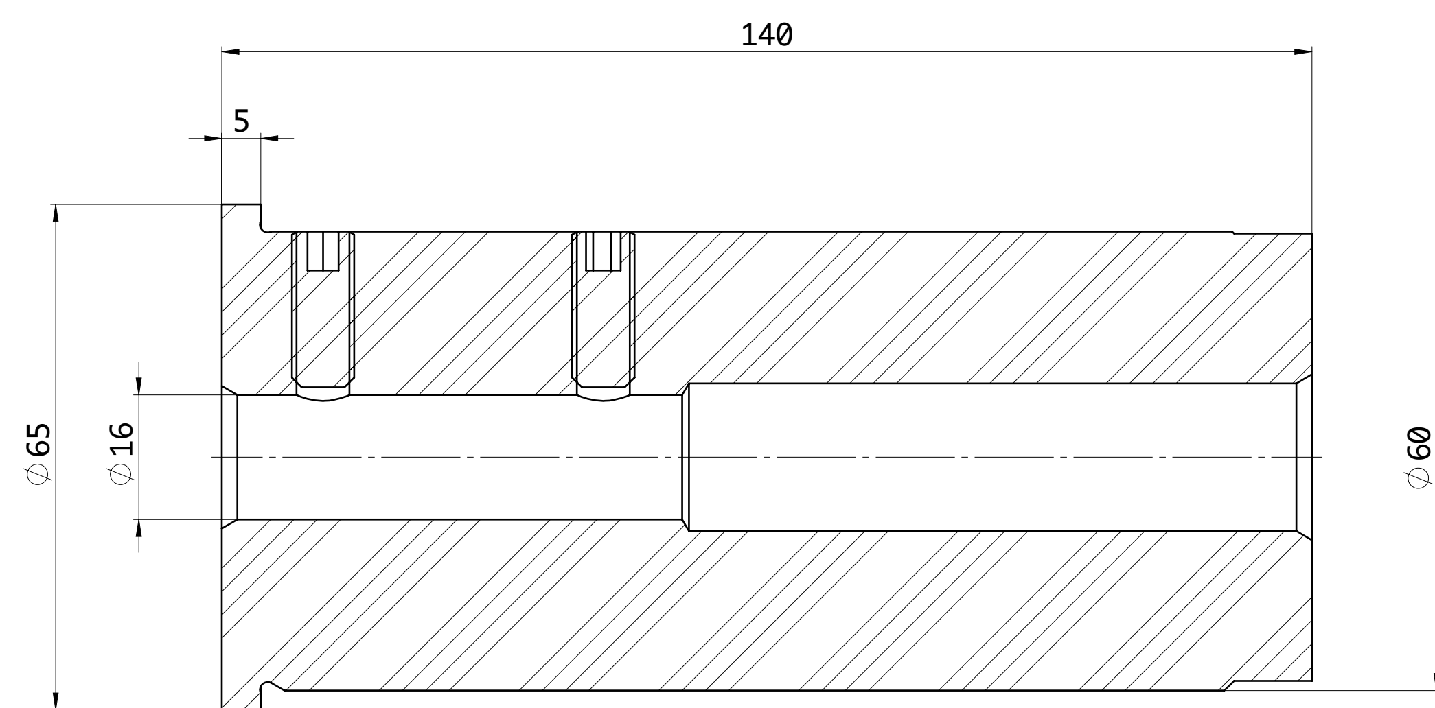
SEZIONE A-A
