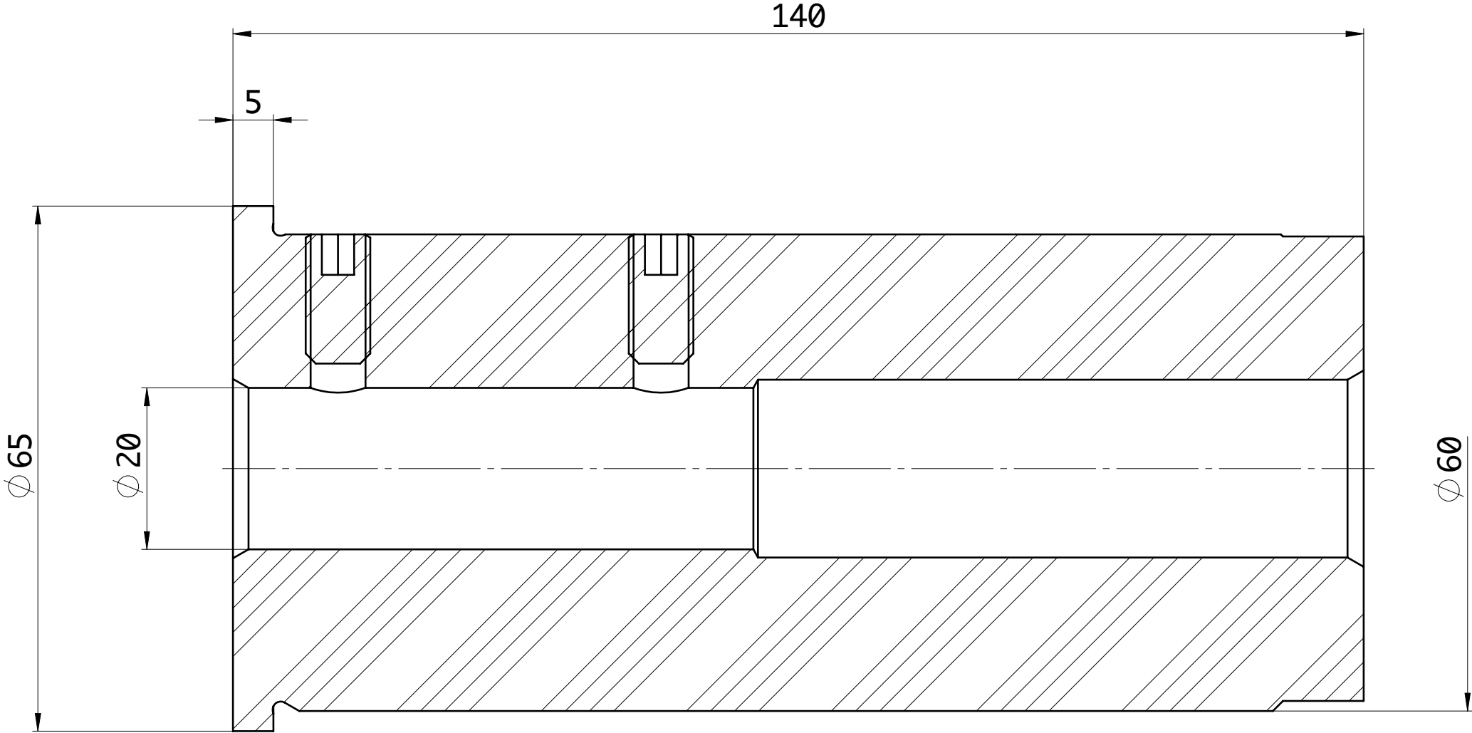
SEZIONE A-A
