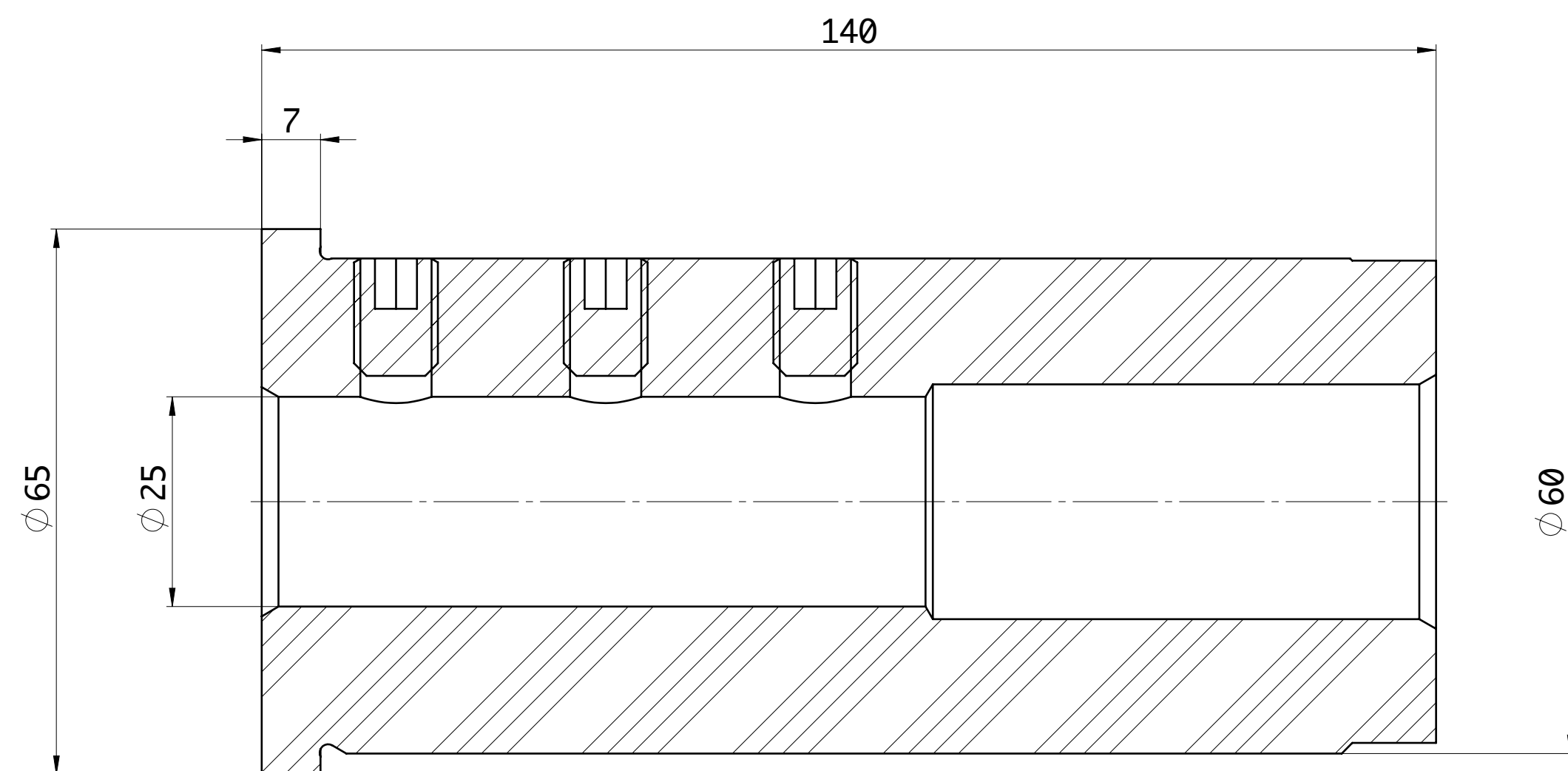
SEZIONE A-A
