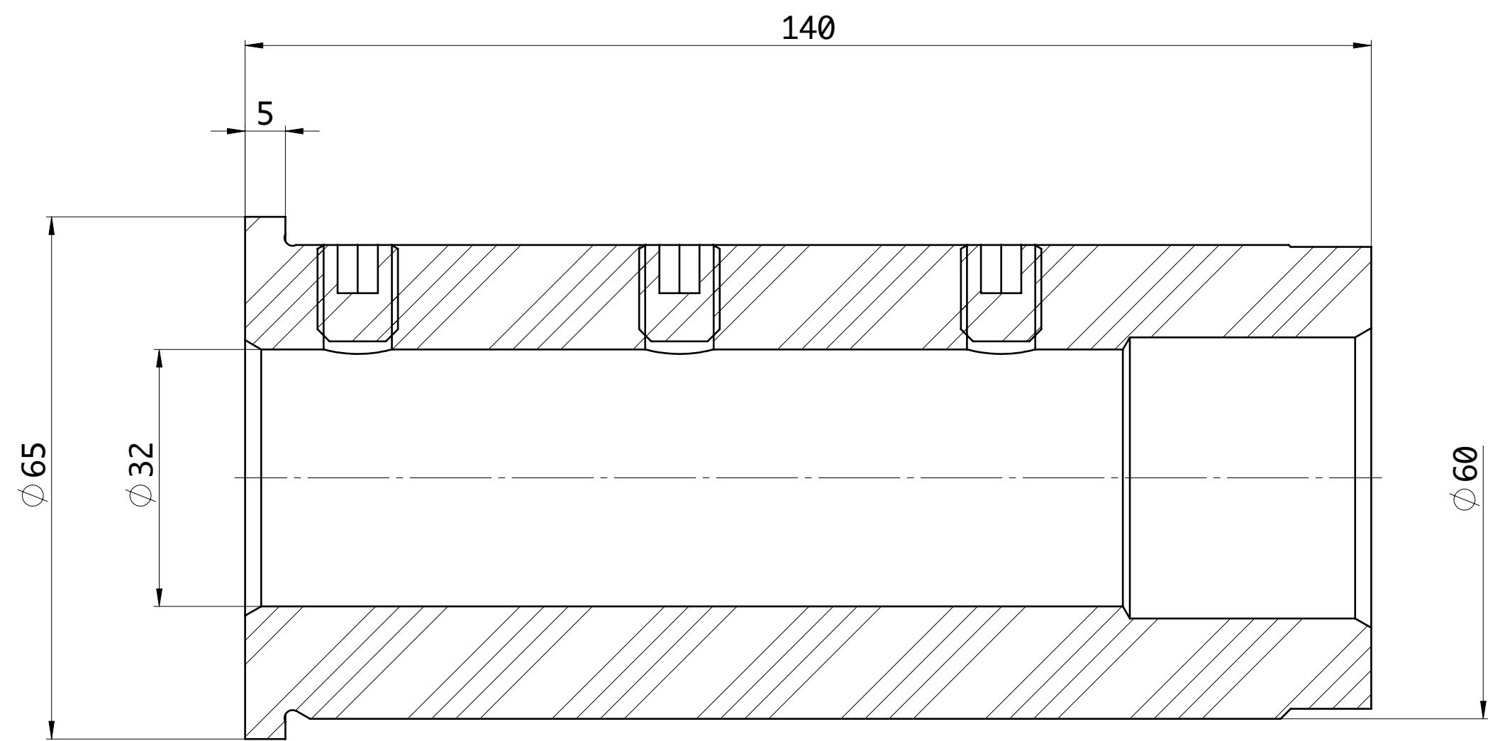
SEZIONE A-A
