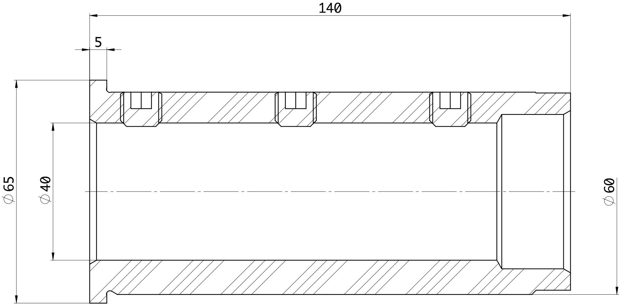
SEZIONE A-A
