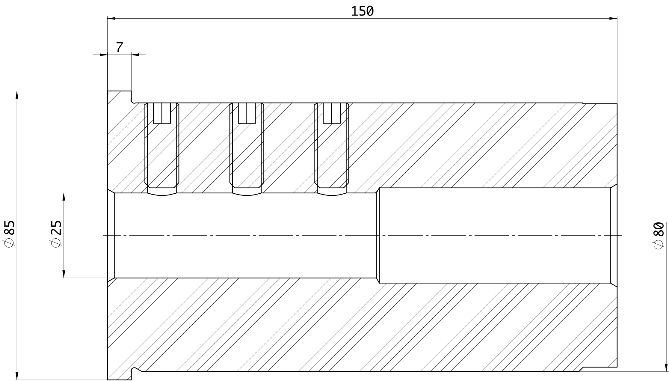
SEZIONE A-A
