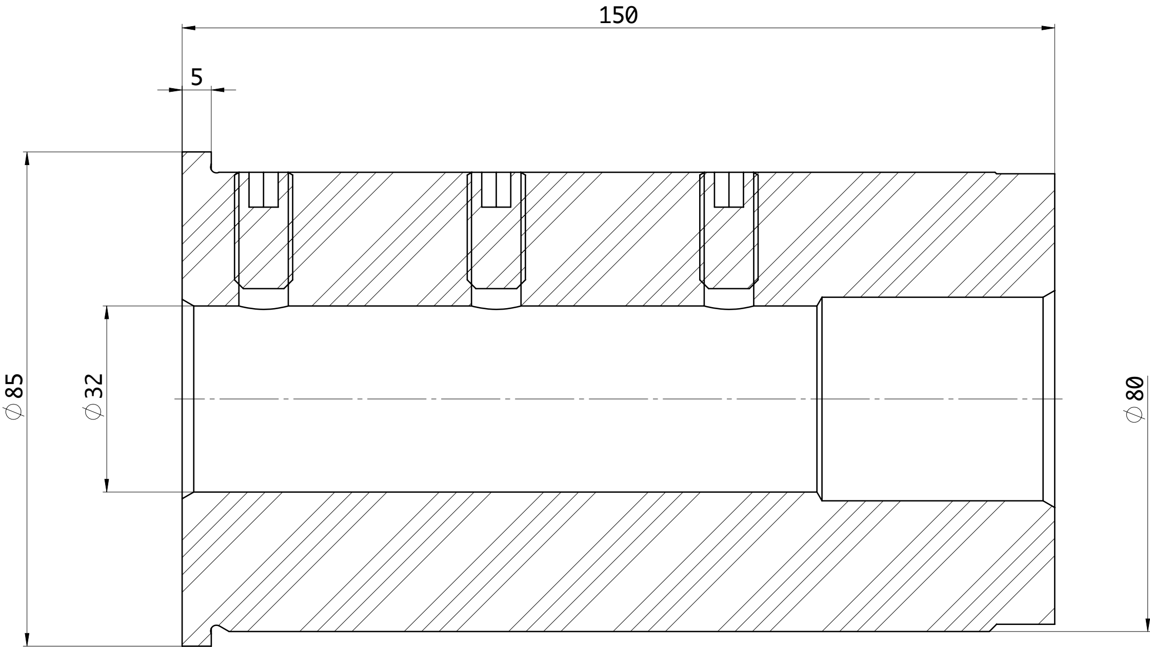
SEZIONE A-A
