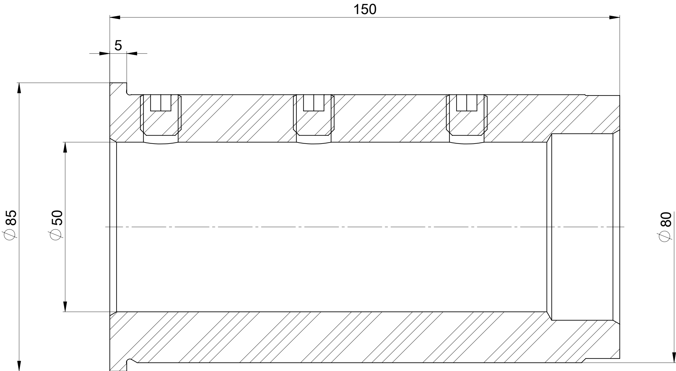
SEZIONE A-A
