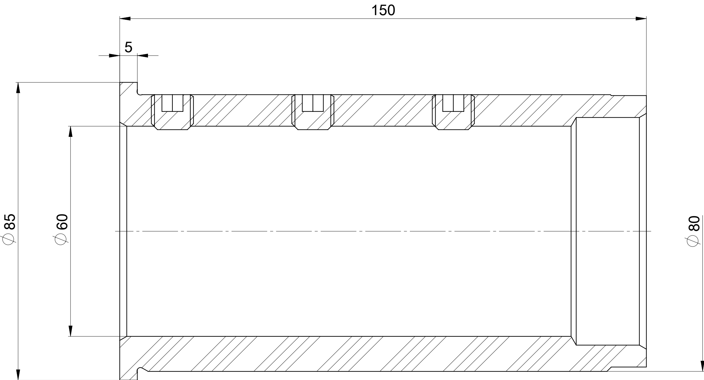
SEZIONE A-A
