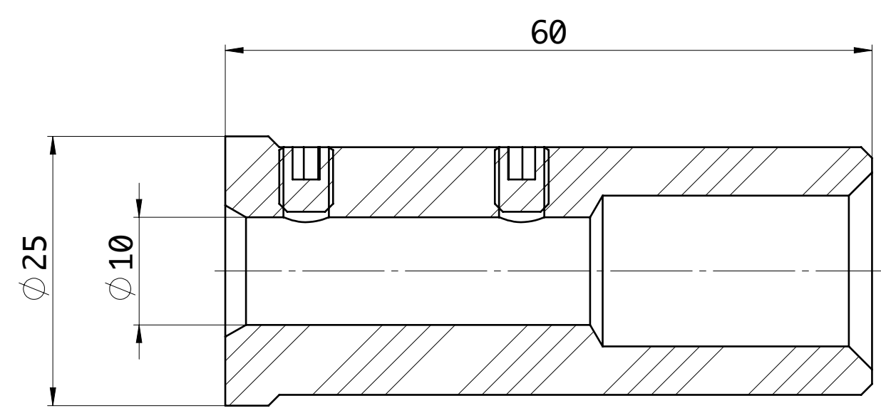
SEZIONE A-A
