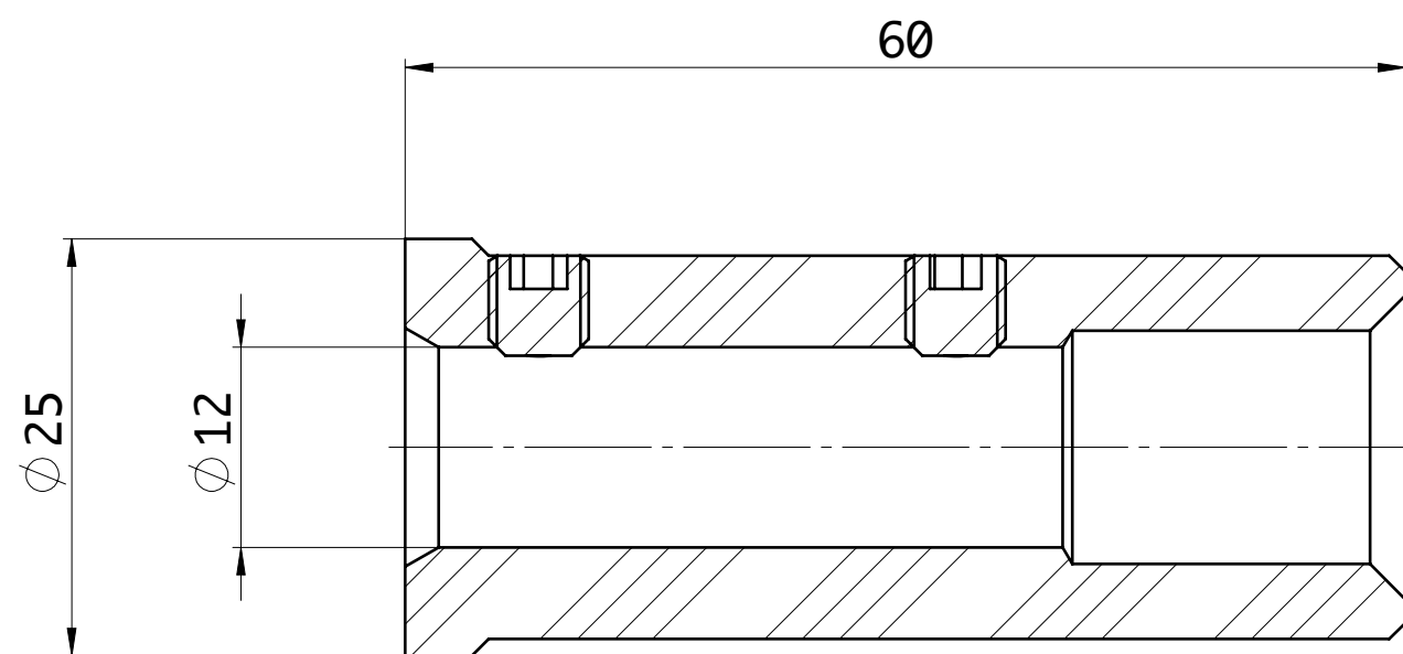
SEZIONE A-A
