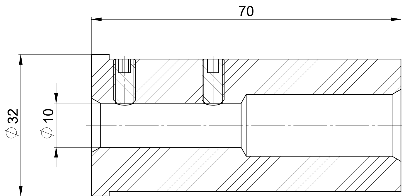
SEZIONE A-A
