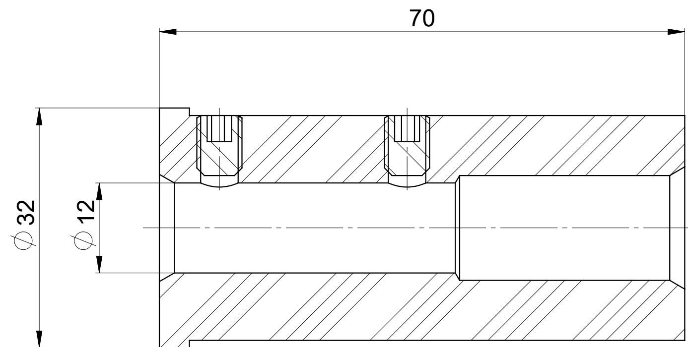
SEZIONE A-A
