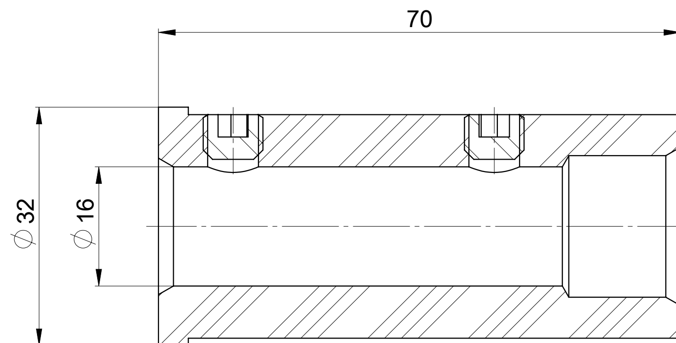
SEZIONE A-A
