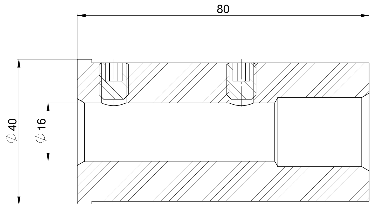
SEZIONE A-A
