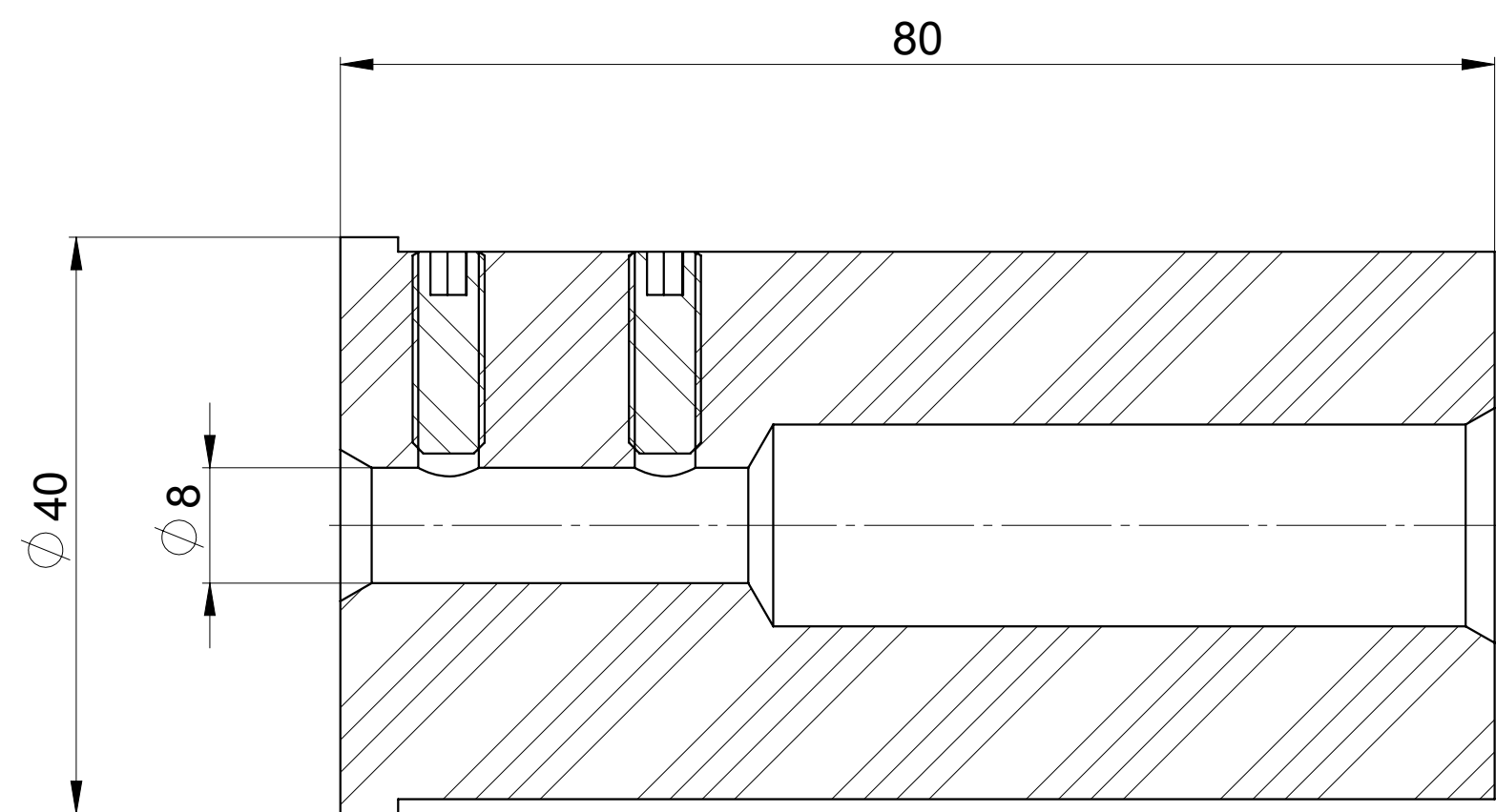
SEZIONE A-A
