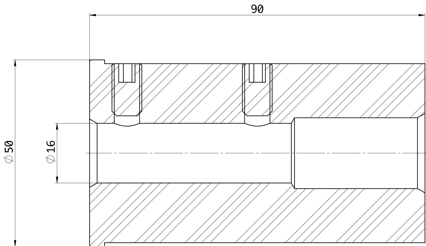
SEZIONE A-A
