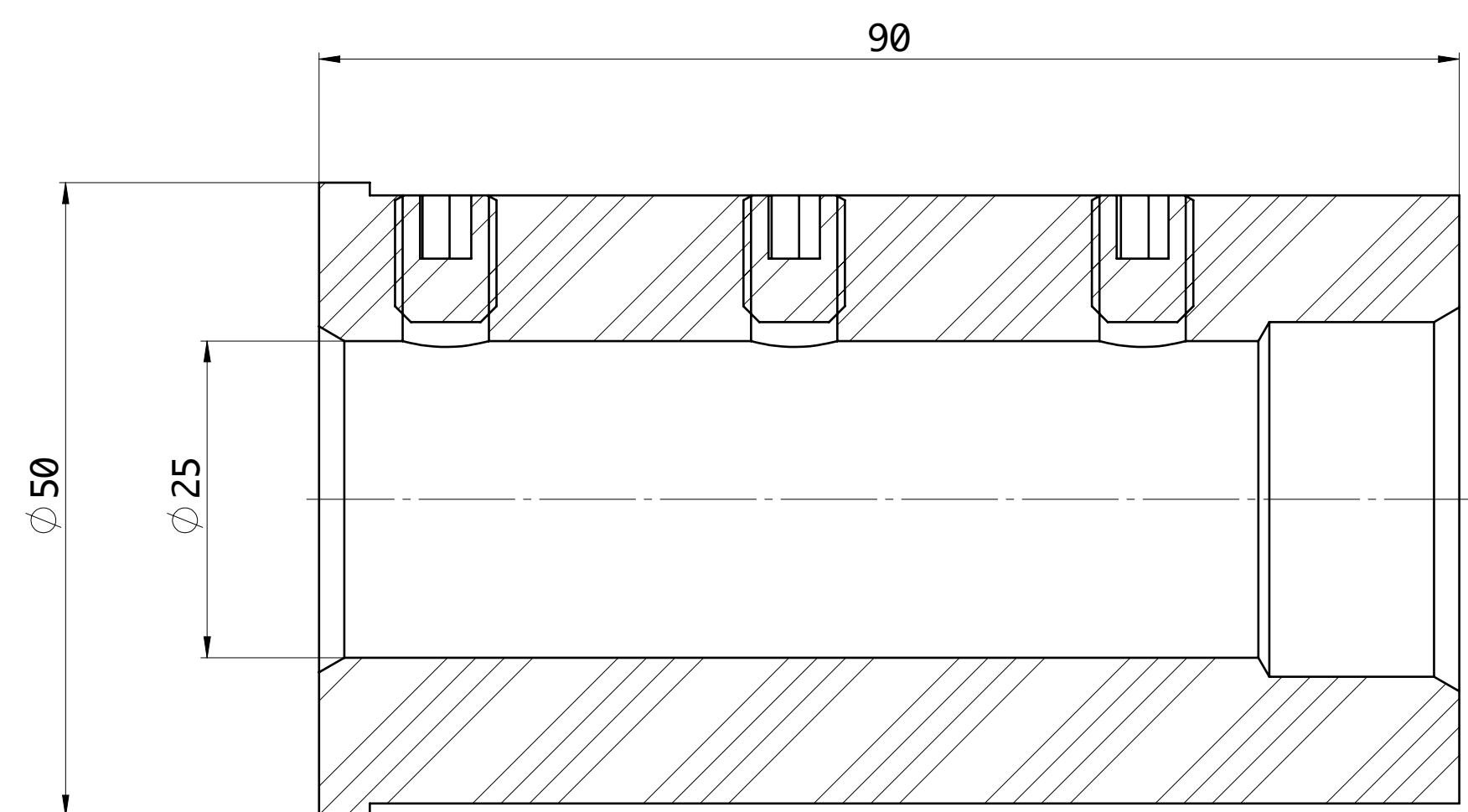
SEZIONE A-A
