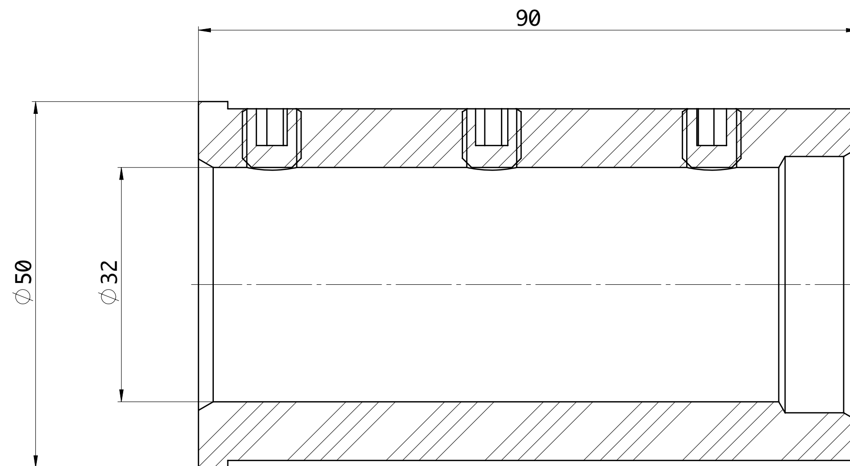
SEZIONE A-A
