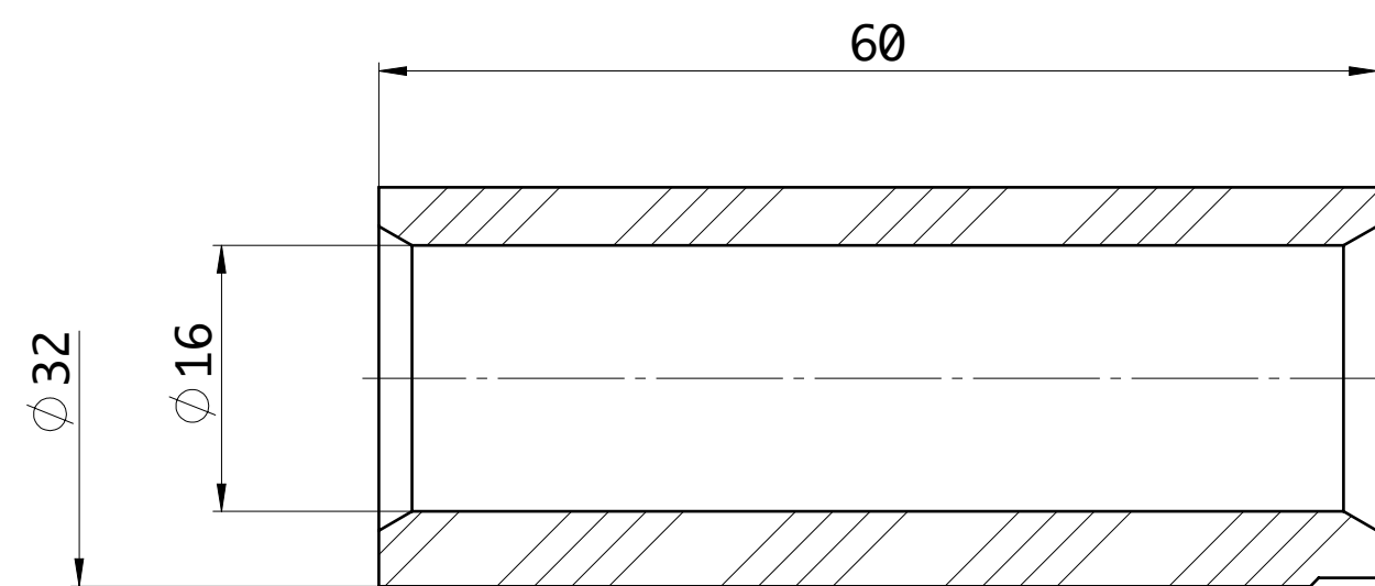
SEZIONE A-A
