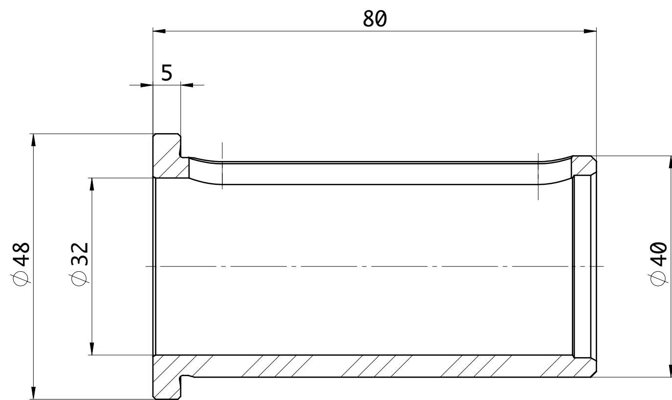
SEZIONE A-A
