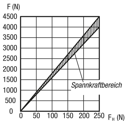
Kräftediagramm
