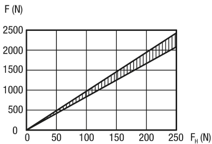
Kräfte diagramm
