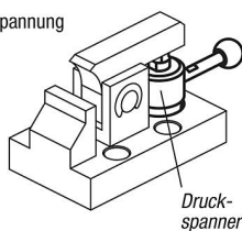
Vertikalspannung
