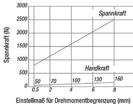
Zugspanner K0910.4050...
