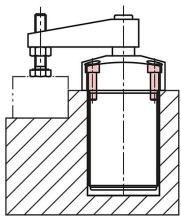
Mit vier Zylinderschrauben von oben.
