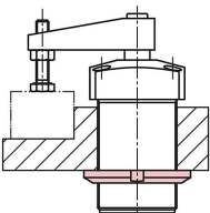
Mit einer Nutmutter von unten.
